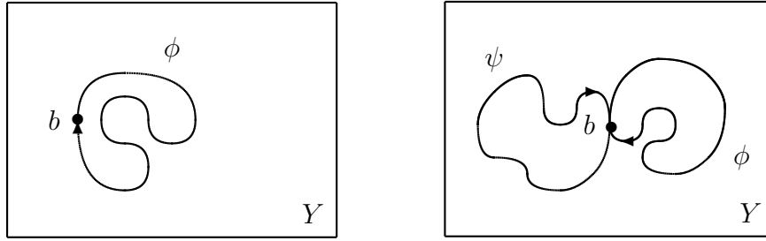
Obrázek 2: Vlevo: typický element prostoru \Omega(Y) . Vpravo: navazování smyček.
