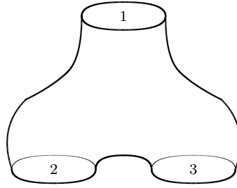
Obrázek 6: Element prostoru \widehat{\mathcal{M}}_0(2) .
