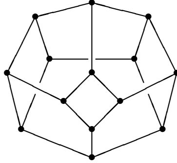
Obrázek 4: Stasheffův asociáedr K_5 .
