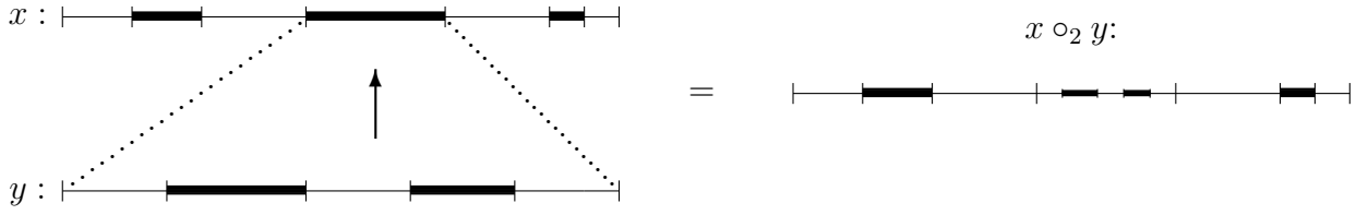
Obrázek 3: Strukturní operace operády malých intervalů. Obrázek naznačuje kompozici x \circ_2 y \in \mathcal{C}_1(4) prvků x \in \mathcal{C}_1(3) a y \in \mathcal{C}_1(2) .
