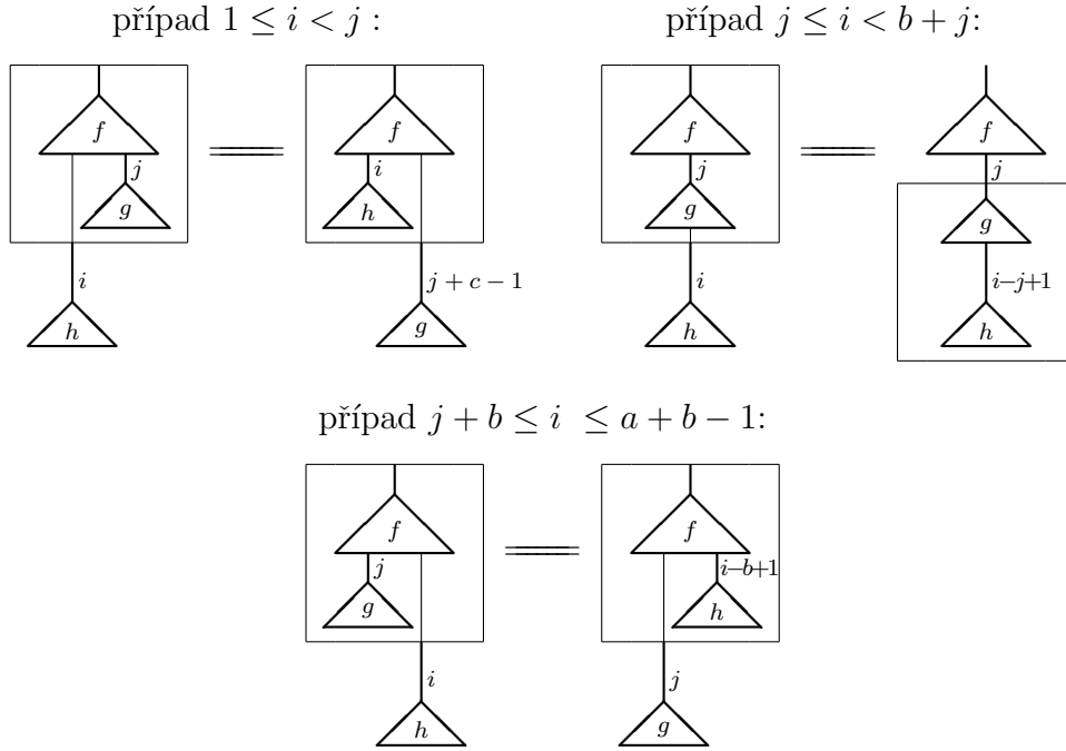
Obrázek 1: Rovnice (3) reprezentovaná „vývojovými diagramy“.
