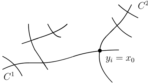
Obrázek 5: Struktura operády \overline{\mathcal{M}} = \{\overline{\mathcal{M}}(n)\}_{n \geq 2} .
